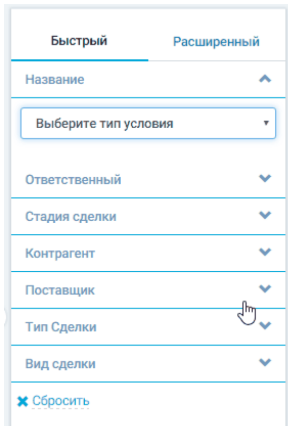
Рисунок 18. Быстрый фильтр
